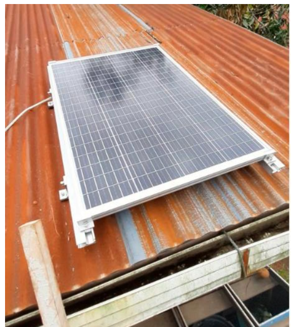
Gambar 6. Pemasangan Panel Surya di Atas Penetasan Telur Itik
